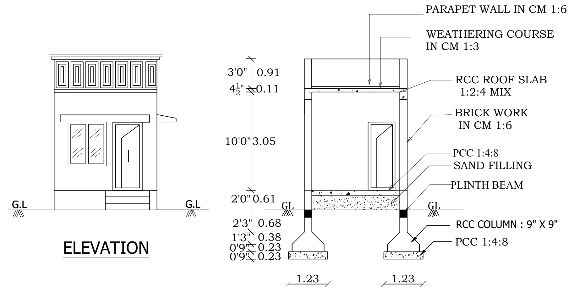
SECTION - AB
