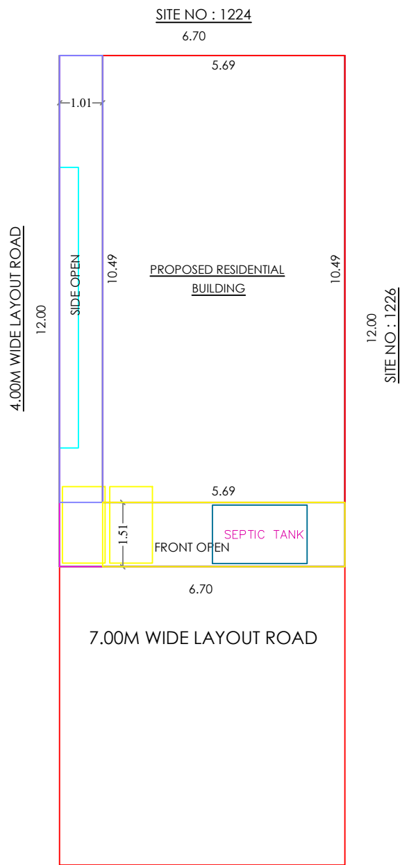
SITE PLAN 1:100
