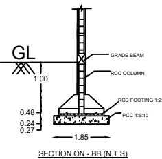
SECTION ON - BB (N.T.S.)
