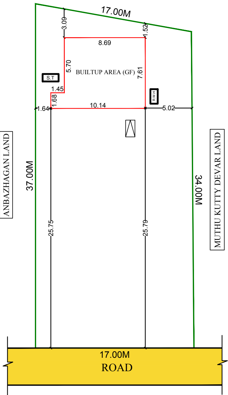
SITE PLAN (1:200)
