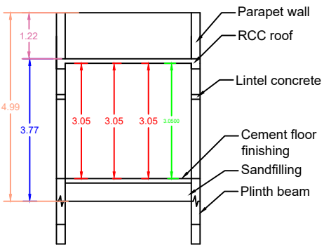
SECTION - AB
