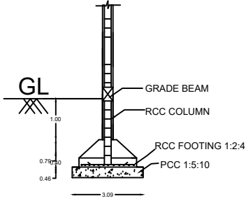
SECTION ON - BB (N.T.S)
