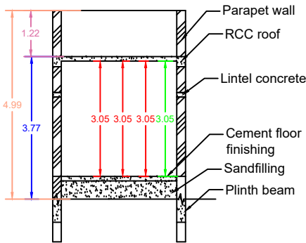
SECTION - AB
