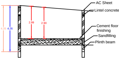
SECTION - AB
