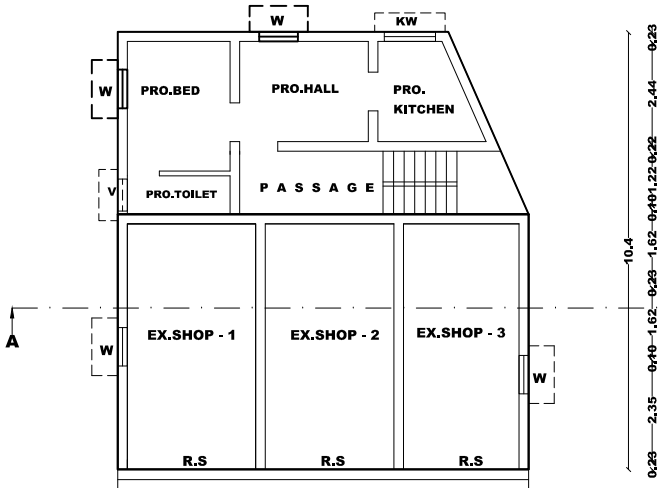
R.W.C.T, PLAN & SECTION
