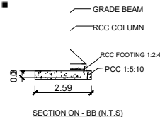
SECTION ON - BB (N.T.S)
