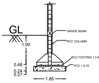
SECTION ON - BB (N.T.S)
