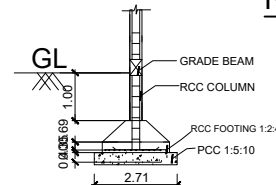
SECTION ON - BB (N.T.S)
