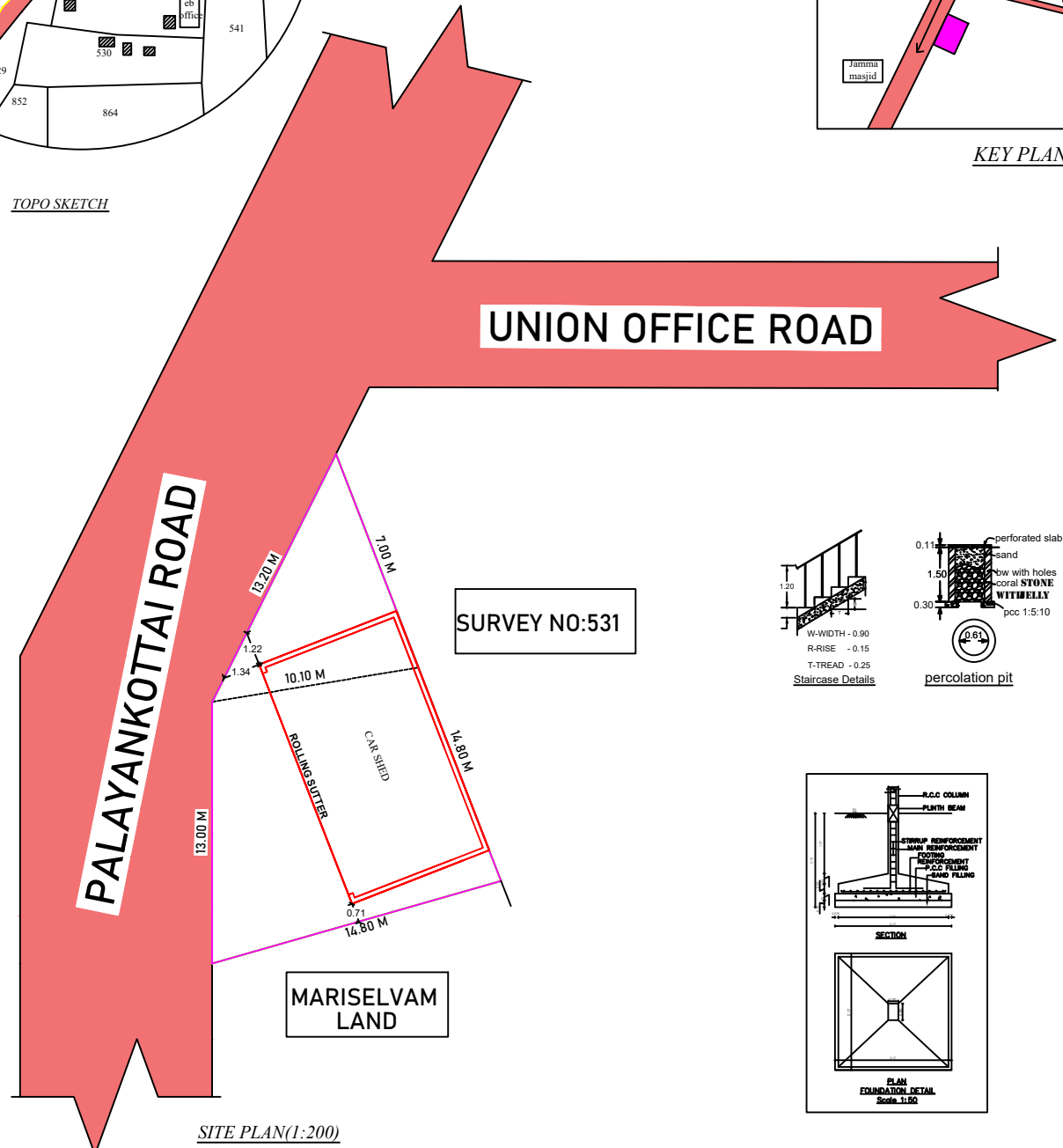
SITE PLAN(1:200)
