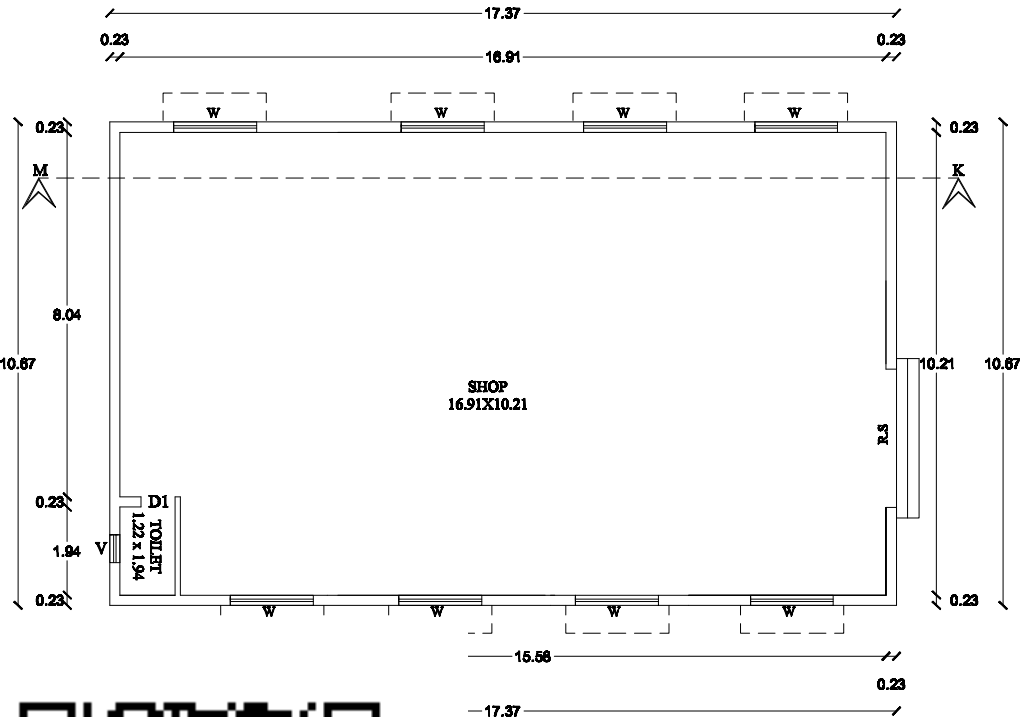
UND FLOOR PLAN
