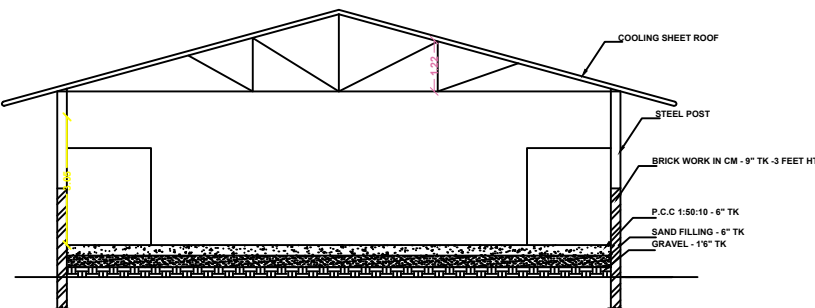
SECTION -AB
