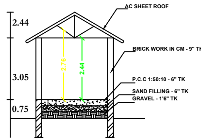
SECTION -AB
