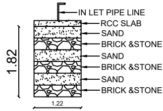
SECTION ON R.W. PITS
