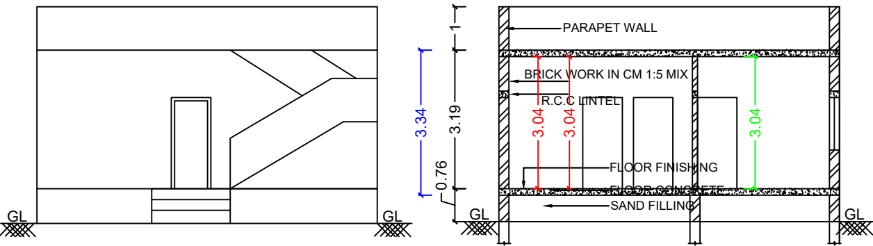
ELEVATION
