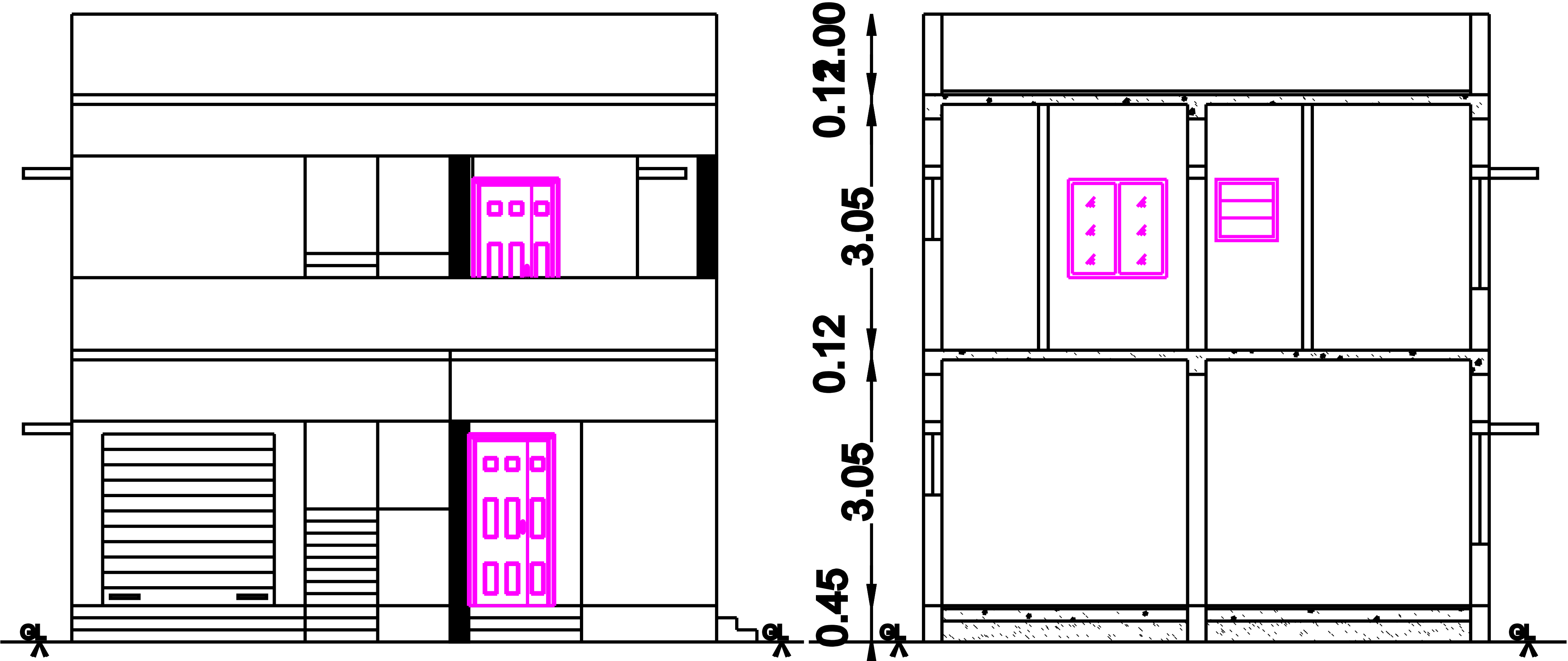
ELEVATION
