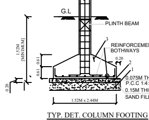
TYP. DET. COLUMN FOOTING
