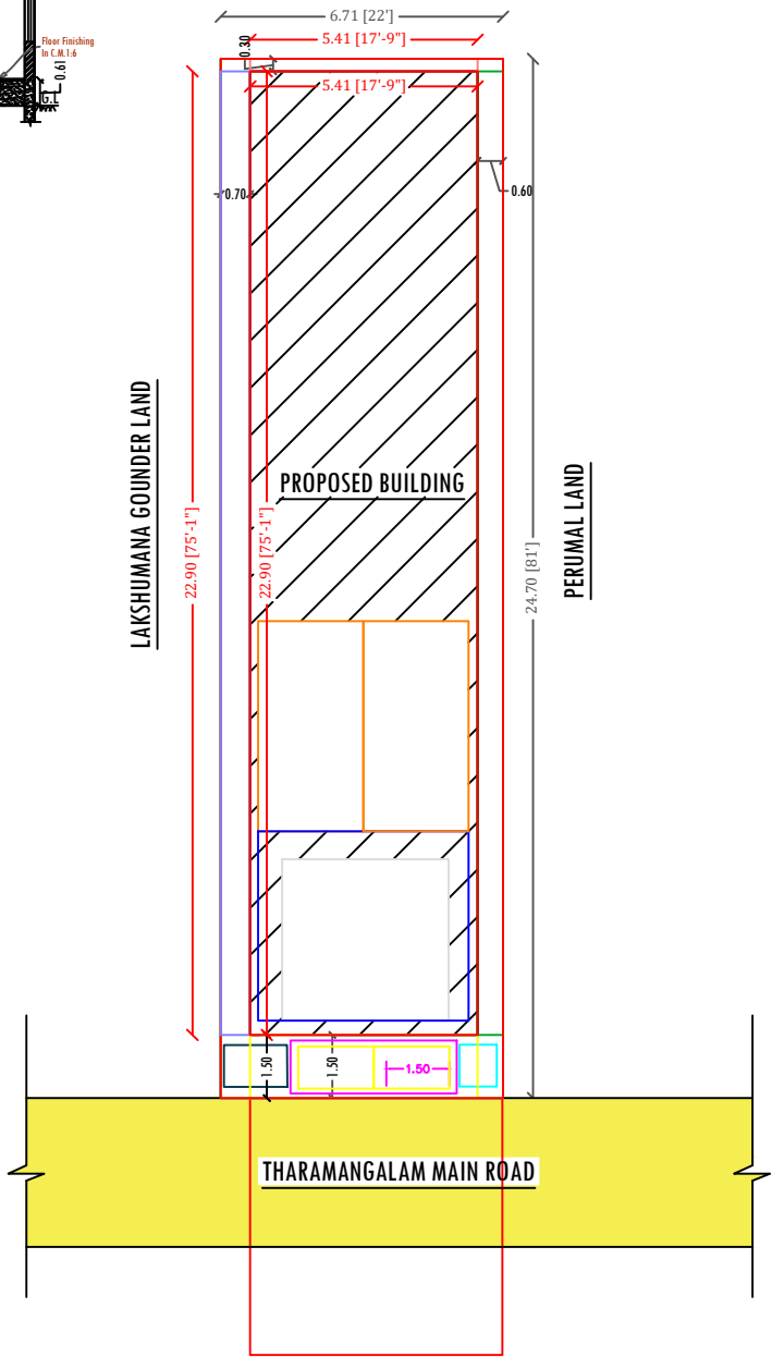
SITE PLAN SCALE - 1:100 PERUMAL LAND
