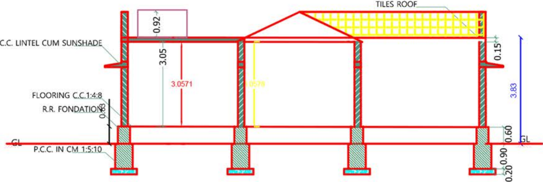
SECTIONN A-A
