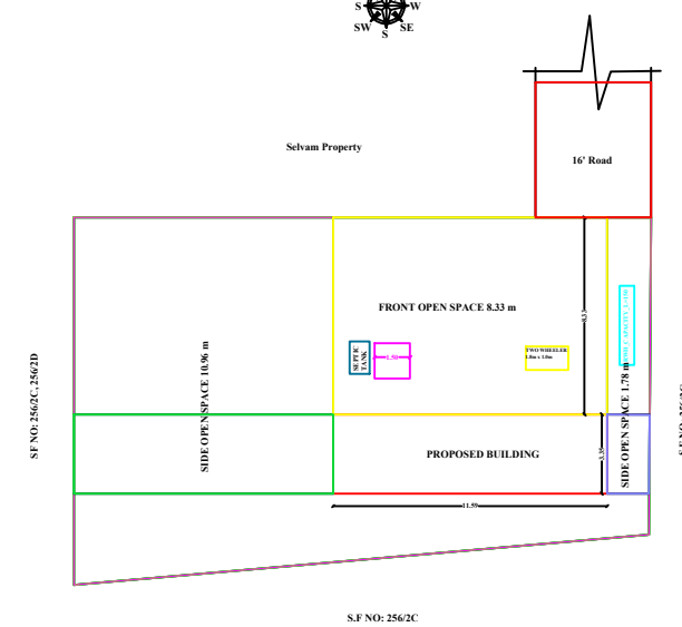
SITE PLAN: SCALE 1:100
