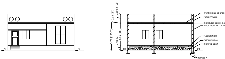
ELEVATION
