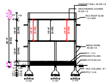
SECTION - AB
