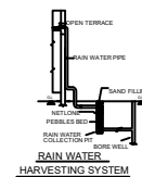
ELEVATION
