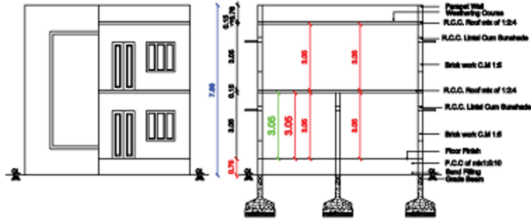
ELEVATION
