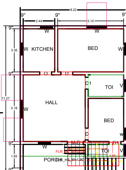
G.F PLAN
