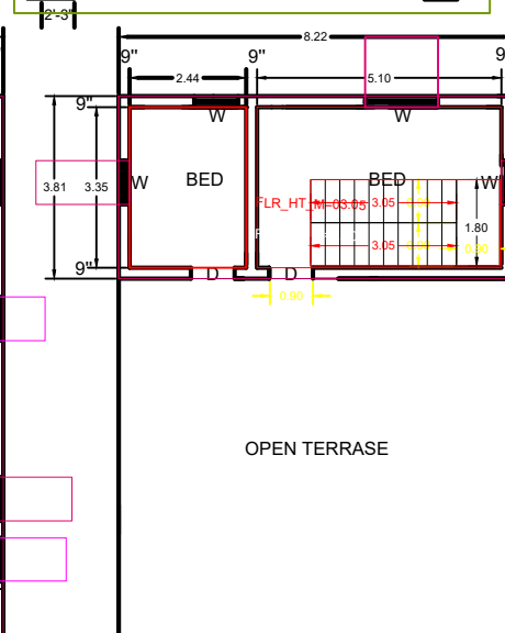
F.F PLAN
